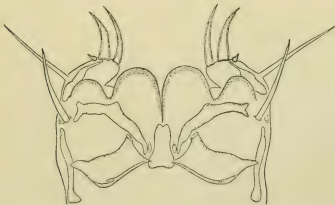
FIG. 25.— Lamippe Duthiersi Joliet. Primer par de patas. X 600.
